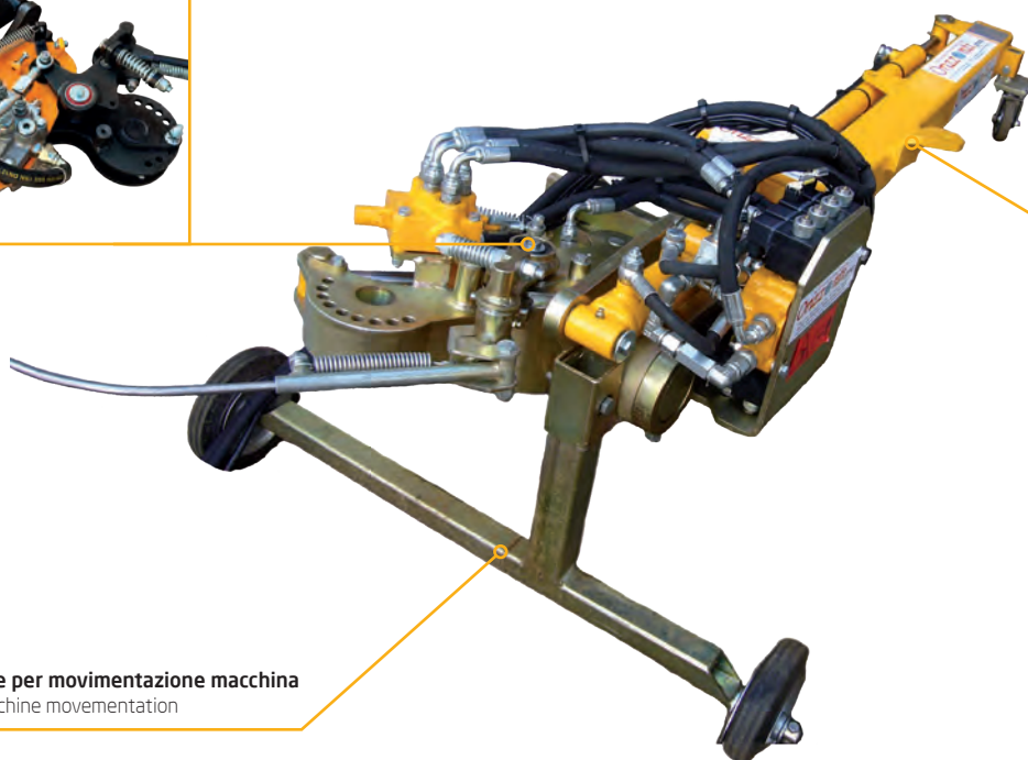
Distributore idraulico 4 leve montato sulla versione 1035200L Hydraulic distributor fix on the 1035200L version.
