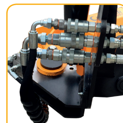
Gruppo innesti rapidi Group of quick connections
