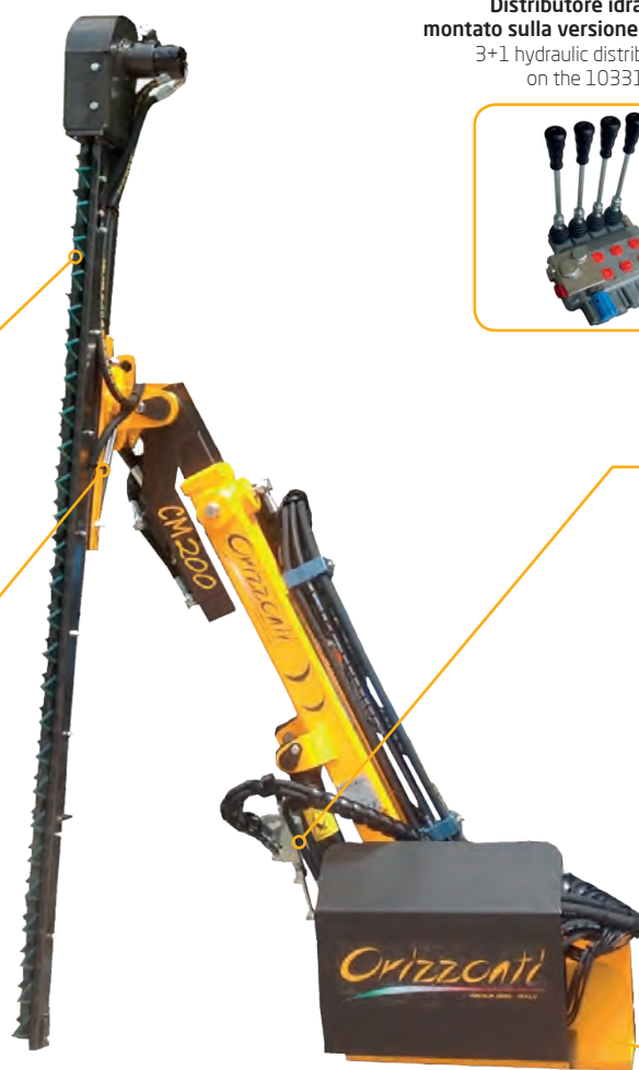
Sistema antiurto barra falciante con molla a gas Mowing bar shockproof system with gas spring
