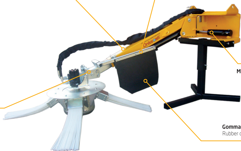
Campana girorami frutteto con regolazione meccanica Pruning rake kit with mechanical adjustment
